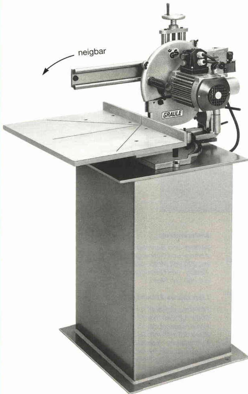
Abläng- und Gehrungskreissäge Typ ZS 85 N
